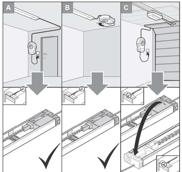
Abb. Einbausituation und die Einbauvarianten A, B und C
