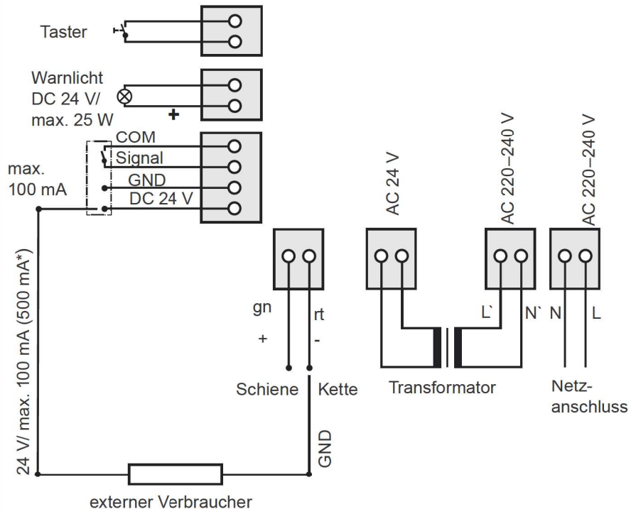
Abb. Anschlussplan Deckensteuerung
